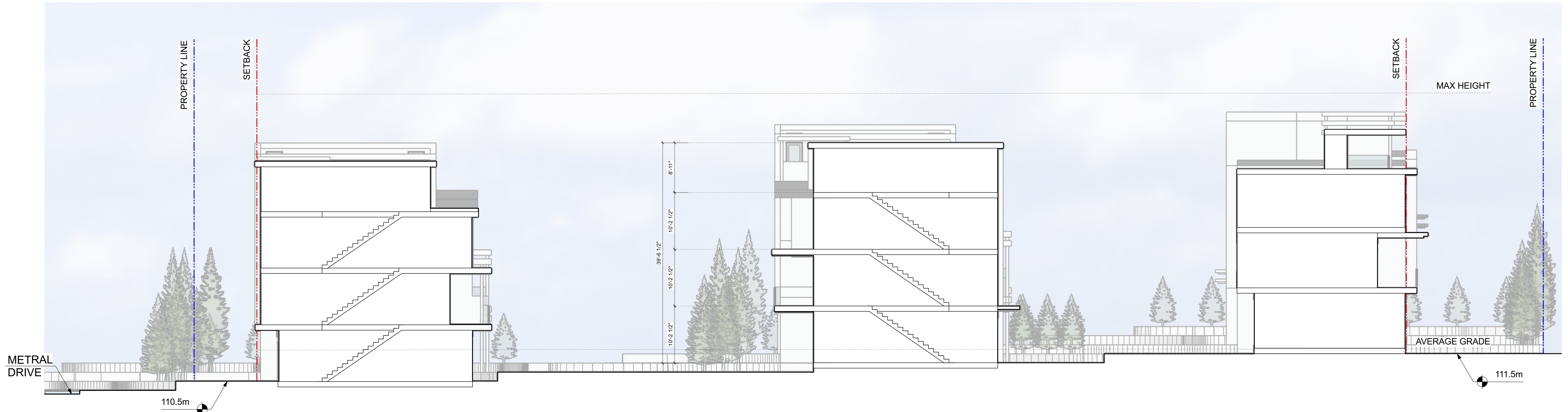
2 Site Section A2 Scale: 1/8" = 1'-0"
